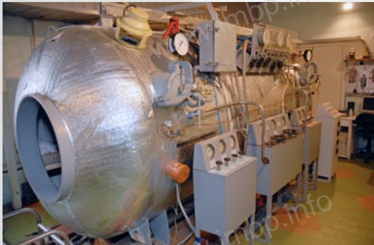
Усовершенствованная поточно-декомпрессионная барокамера ПДК-2 УМ Upgraded continuous-decompression chamber PDK-2 UM
